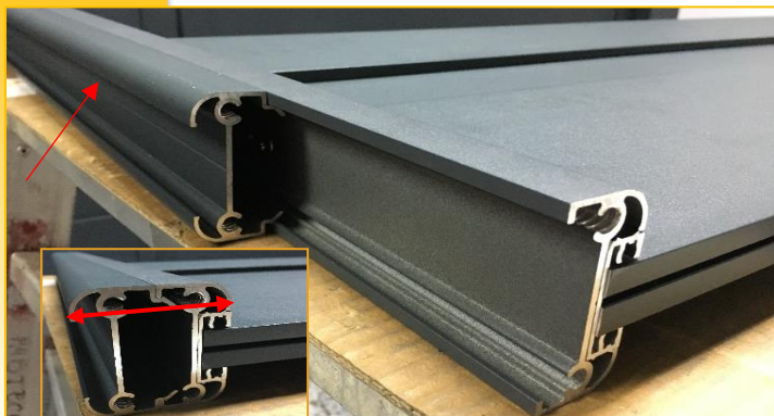
Demi-potelet d'extrémité ajouté au demi-potelet intermédiaire du module de clôture. Les 2 forment un poteau complet d'environ 60 mm.
