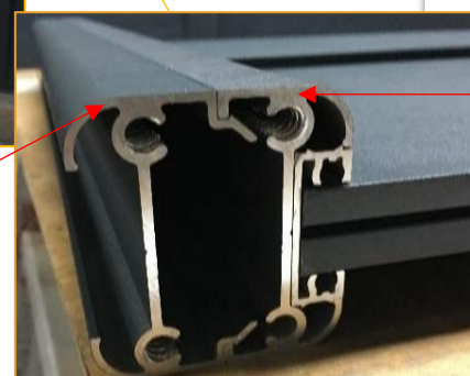
demi-potelet d'extrémité mâle avec encoches
